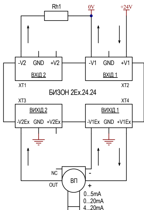
Струмова петля 0-5 мА, 0-20 мА, 4-20 мА (2-провідне підключення)
