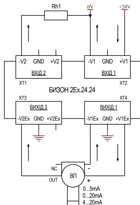
Струмова петля 0-5 мА, 0-20 мА, 4-20 мА (3-провідне підключення)
